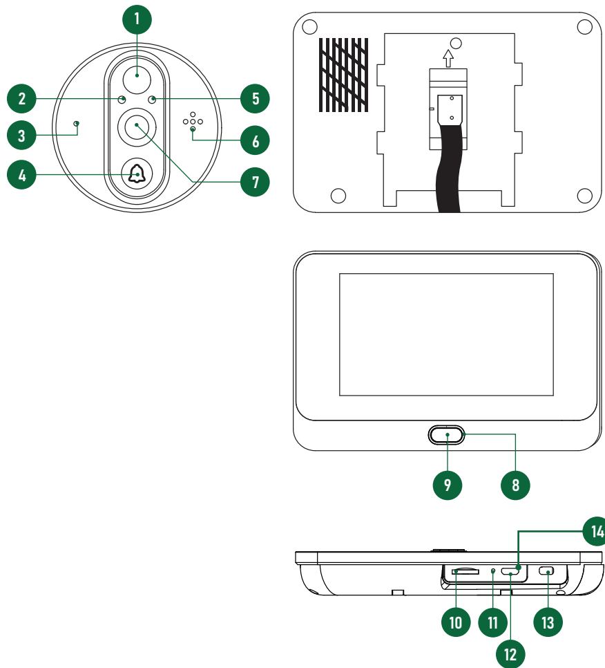
Рис.2 Описание видеоглазка FOCUS 4 WIFI KIT
