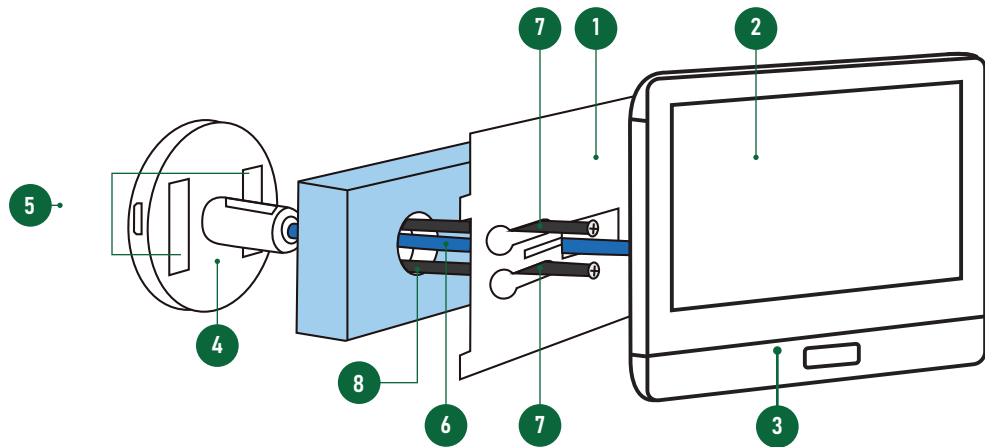
Рис.3 Установка видеоглазка
