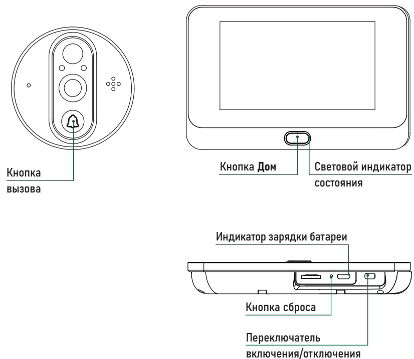
Рис.6 Элементы управления и индикации
